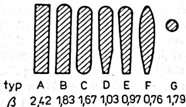
Obr. 23 Tvary průřezů česlic a jejich součinitele \beta [14]
