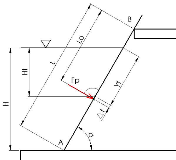
Obr. 24 Tlaková síla
