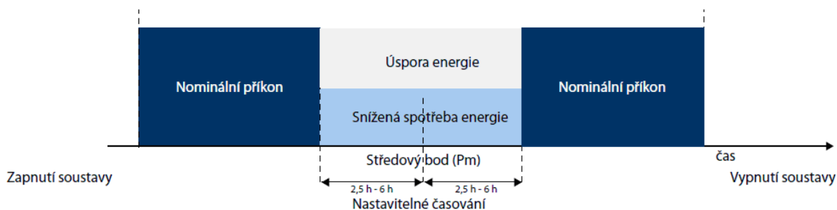
Obrázek 8-13: Možnosti redukce výkonu pomocí elektronického předřadníku ECOLUM [17].
