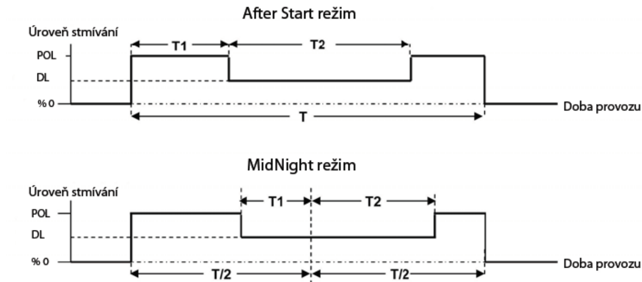
Obrázek 8-10: Ukázka provozních režimů stmívacího systému EHID [20].
