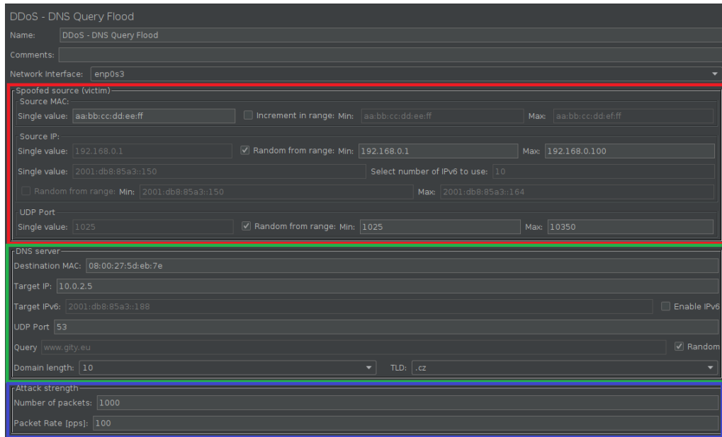
Obr. 2.1: Uživatelské rozhraní DNS Query Flood.
