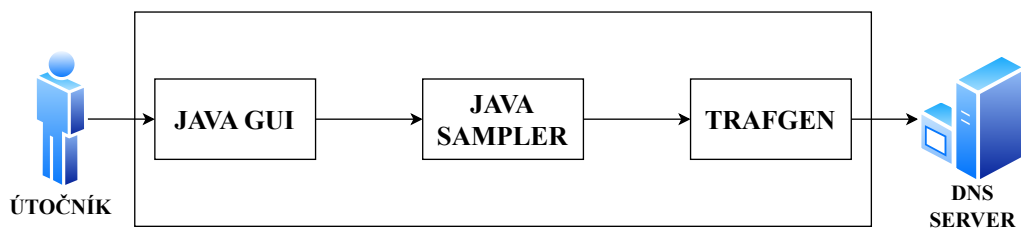
Obr. 2.2: Diagram průběhu útoku.
