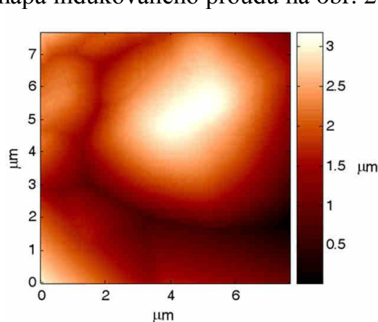
Obr. 19: Topografie vzorku s pyramidální texturou povrchu.
