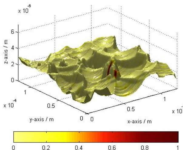
Obr. 23: Obraz lokálního vyzařování namapovaný na topografii vzorku.
