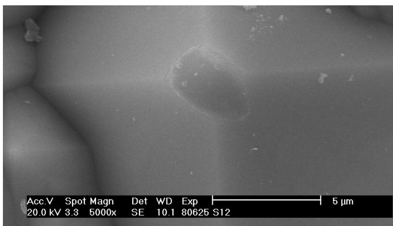
Obr. 28: SEM defektu solárního článku.
