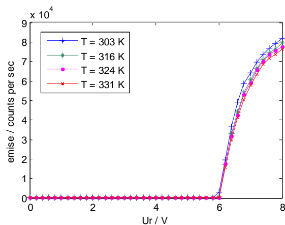
Obr. 9: Závislost vyzařování defektu na závěrném napětí.
