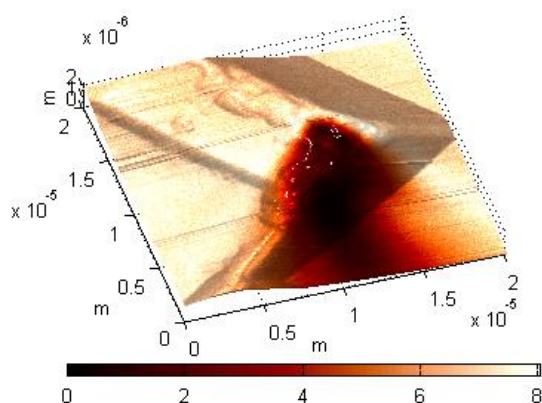
Obr. 25: Relativní mapa stínu hrotu mapovaná na topografii, U_r = 10 V.
