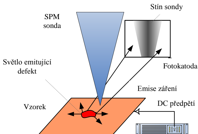
Obr. 21: Princip mikroskopické lokalizace vyzařující nehomogenity.
