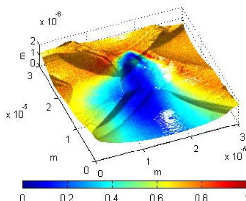
Obr. 31: Relativní mapa stínu hrotu mapovaná na topografii U_r = 21 V.
