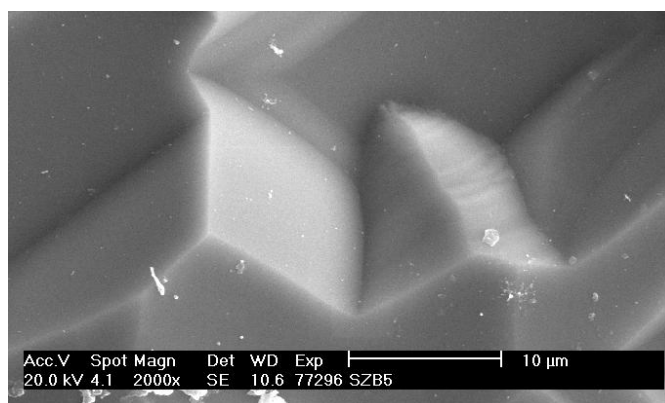
Obr. 27: SEM oblasti solárního článku s defektní morfologií.
