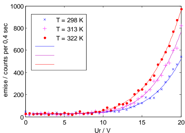
Obr. 14: Závislost emise z hrany opracované pilou na závěrném napětí.
