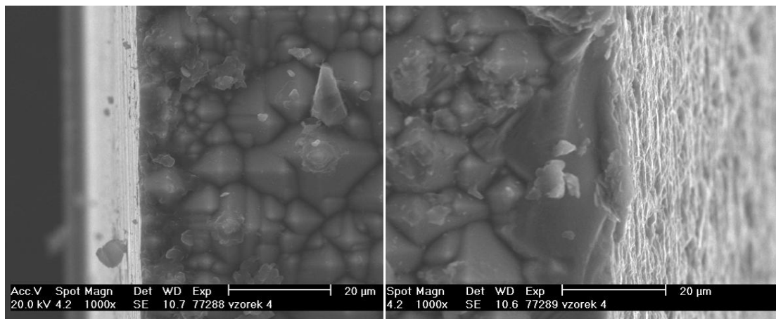
Obr. 15: SEM hrana vytvořená čistě lomem vlevo a obráběním vpravo.
