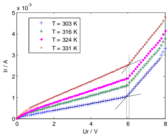
Obr. 8: VA charakteristiky vzorku s výrazným objemovým defektem.
