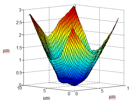
Obr. 17: Určený tvar zkreslujícího hrotu.
