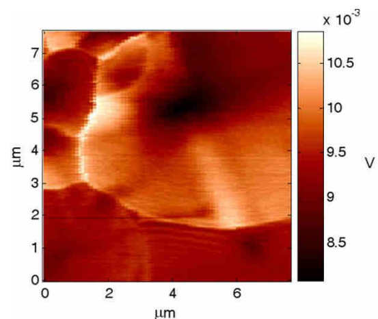
Obr. 20: Obrázek světlem indukovaného proudu.
