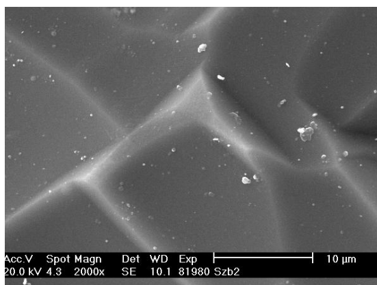
Obr. 30: SEM povrchu vzorku v oblasti lokalizované světelné emise.
