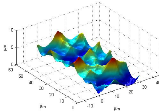
Obr. 18: Rekonstruovaný povrch solárního článku s využitím obálkové metody.
