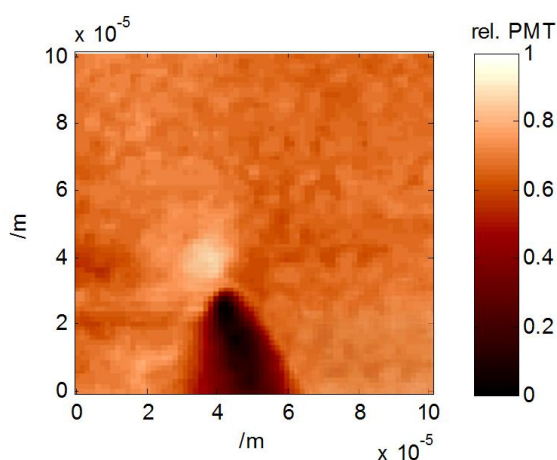
Obr. 22: Stínová mapa světlo emitujícího defektu.
