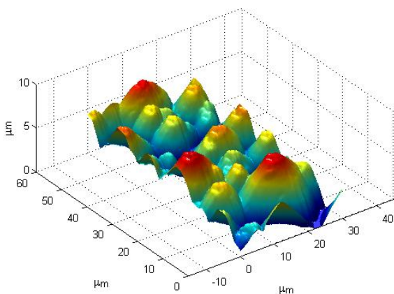
Obr. 16: Naskenovaný povrch solárního článku (poškozený hrot).
