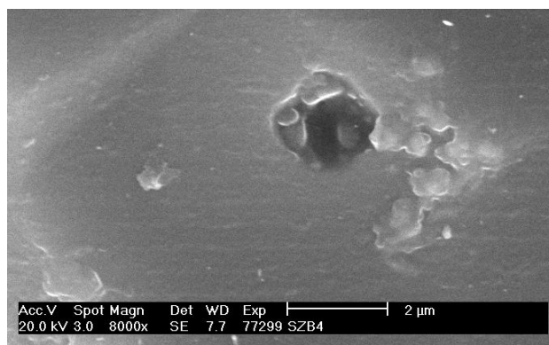
Obr. 24: SEM defektu vykazujícího emisi při U_r = 3 \text{ V} , T = 304 \text{ K} .
