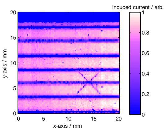
Obr. 10: LBIC části solárního článku s mikrotrhlinami.
