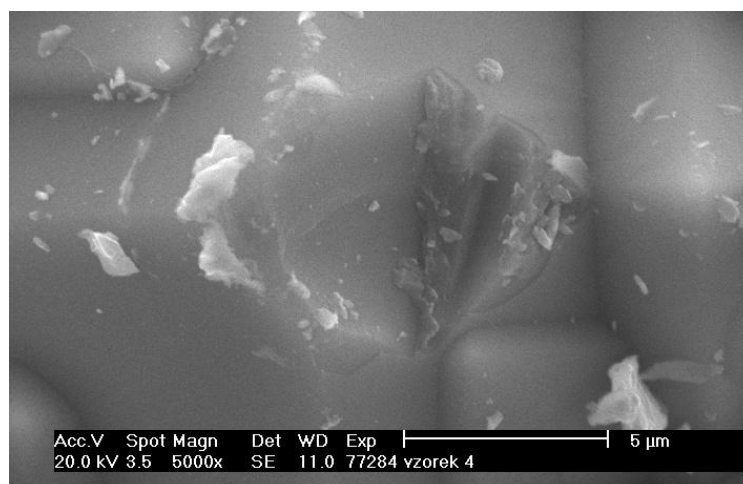
Obr. 29: SEM mechanicky poškozeného povrchu solárního článku.
