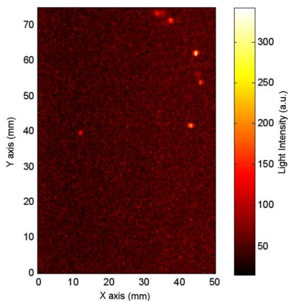
Obr. 6: Emise při závěrné polarizaci přechodu, závěrné napětí U_r = 3,7 \text{ V} .
