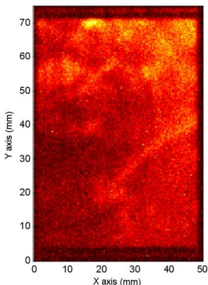
Obr. 5: Emise při propustné polarizaci přechodu, U_f = 1,3 \text{ V} .
