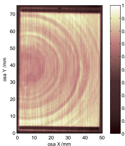
Obr. 3: Relativní mapa LBIV, nehomogenita substrátu.
