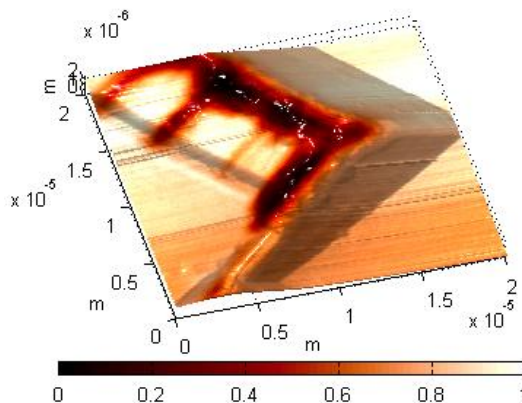
Obr. 26: Relativní LBIC mapovaný na topografii.
