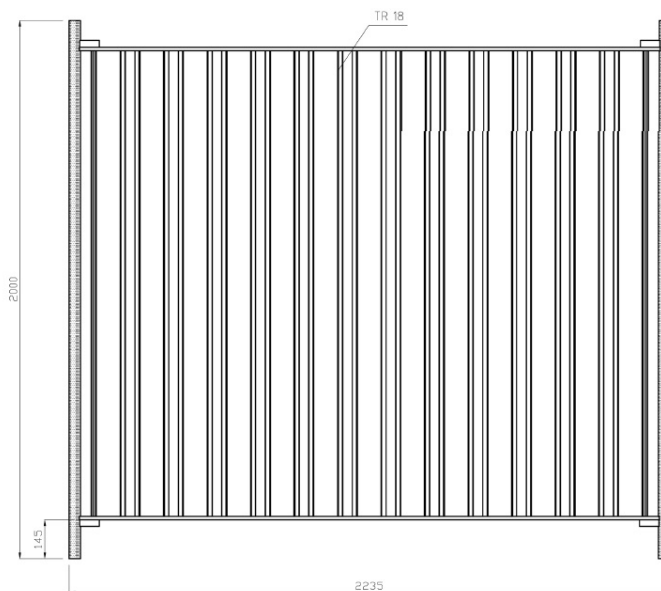
Obr. 25 Mobilní oplocení
