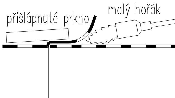
Obr. 20 Svařování přesahů kaširovaných dílců
