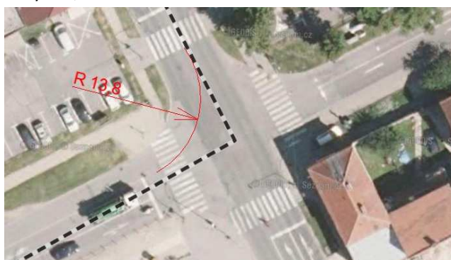
Obr. 12 Kritické místo C
