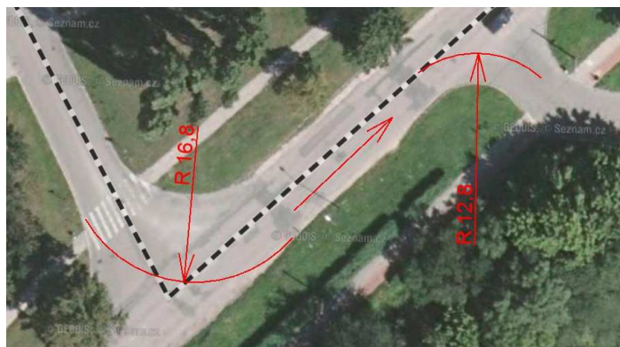
Obr. 18 Kritická místa D, E
