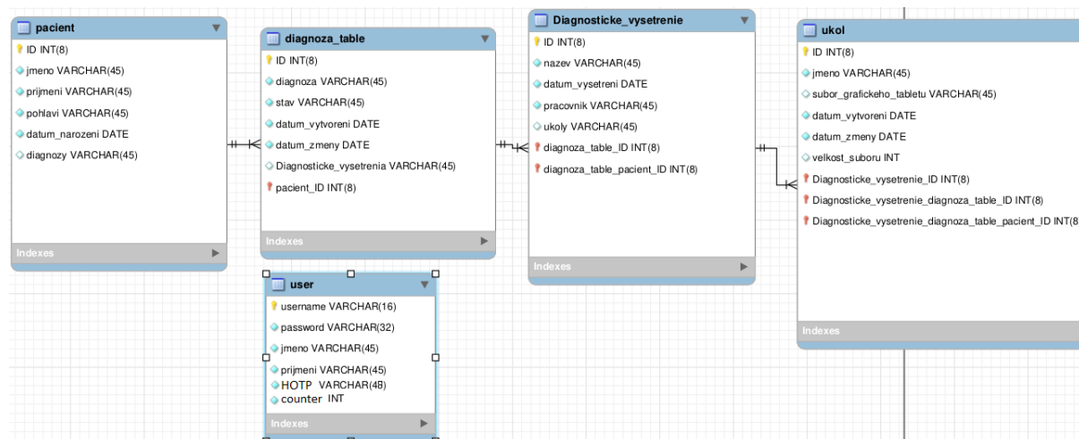
Obr. 4.2: Model databáze
