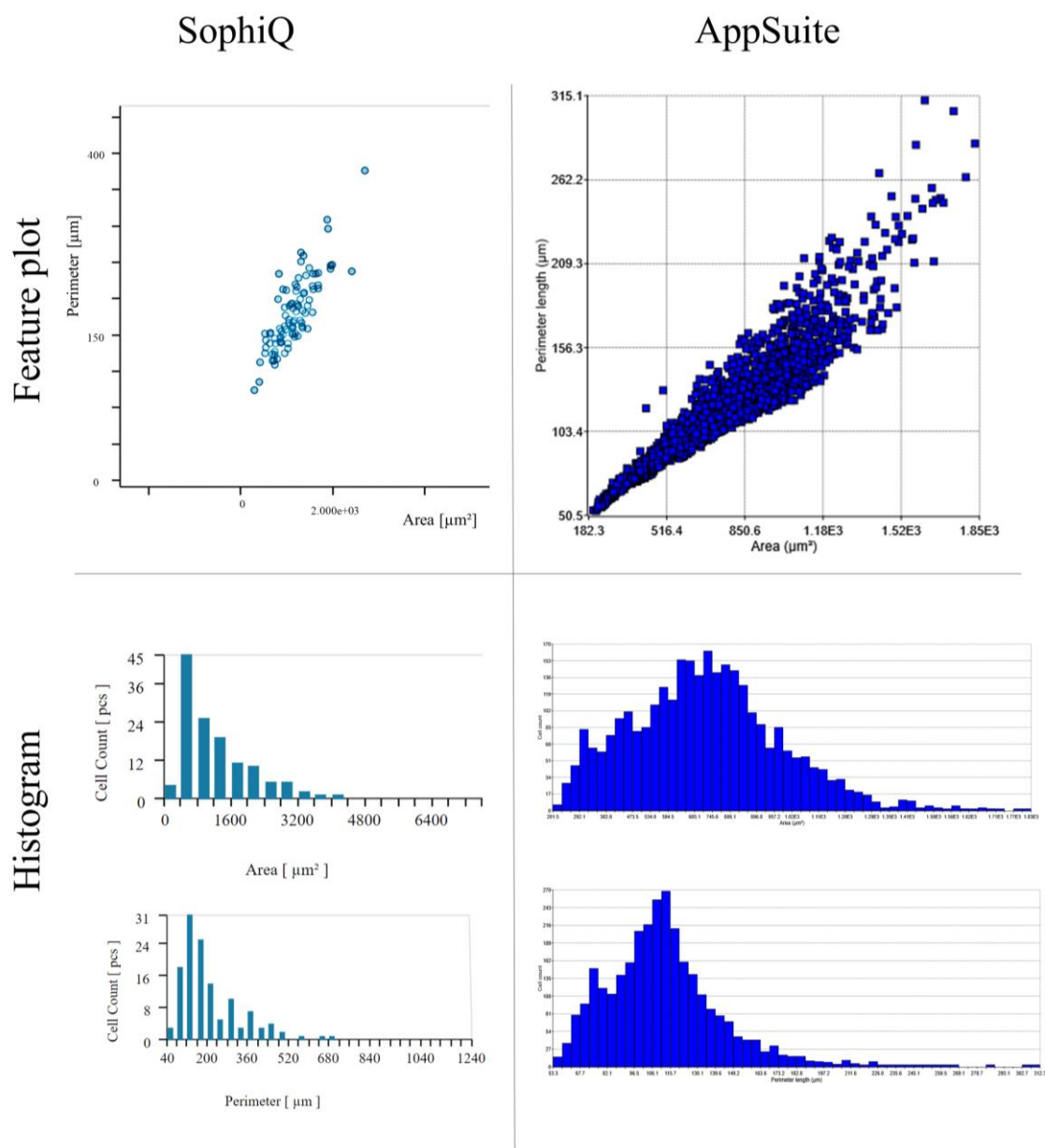
Obrázek č. 39: Srovnání výstupů ze softwarů SophiQ a App Suite. V horní části jsou zobrazeny tzv. feature plot. SophiQ ukazuje hodnoty buněk, které jsou analyzovány v konkrétním časovém úseku. App Suite ukazuje hodnoty všech analyzovaných buněk za celý časový úsek měření. Proto je na grafu z App Suite zobrazeno více hodnot. Obou případech se jedná o ukázkou, kdy na ose x jsou hodnoty areí a na ose y perimetru buněk. Spodní grafy představují histogramy parametrů areí a perimetru na konci měření.
