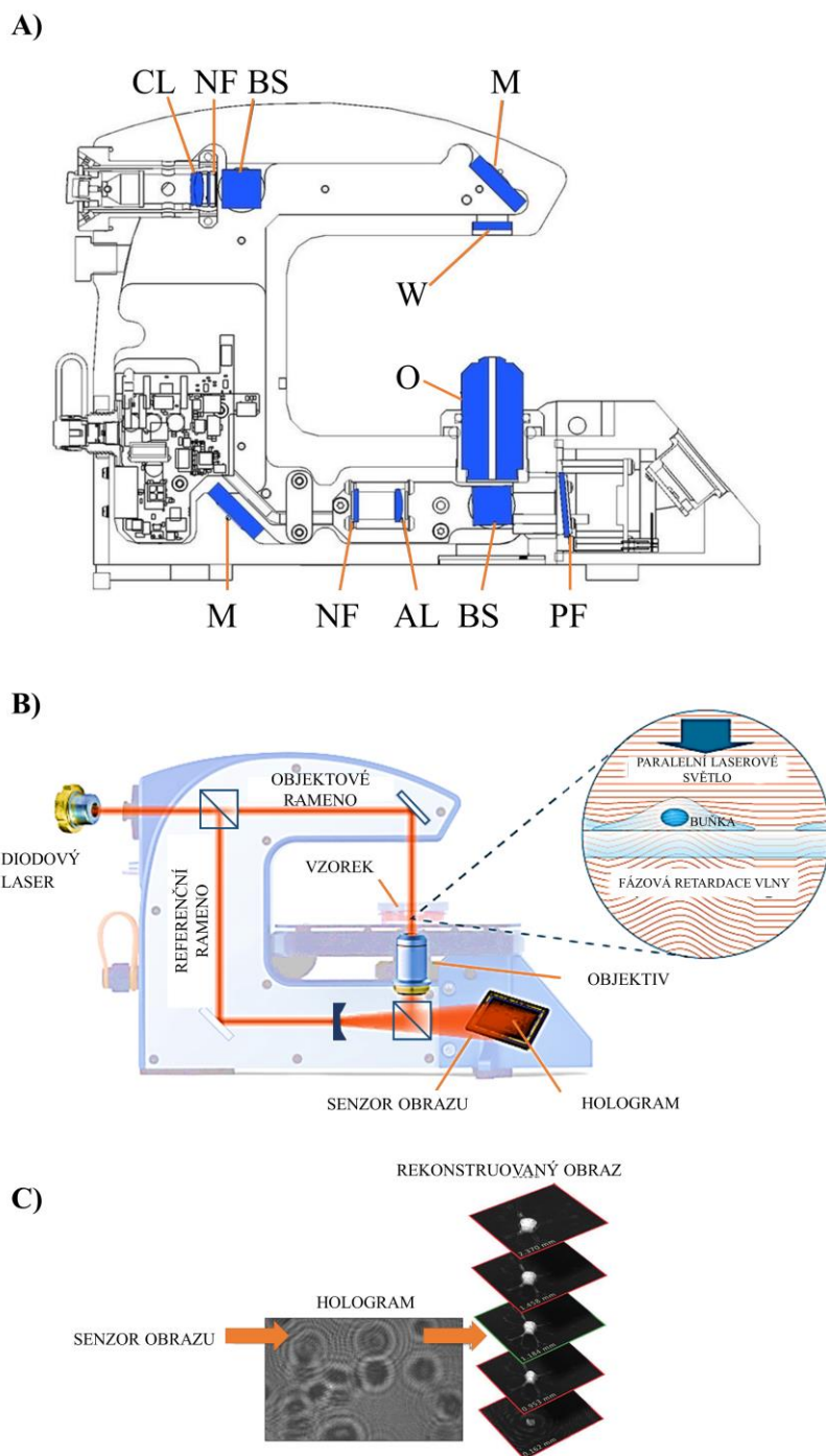
Obrázek č. 34: Optické schéma holografického mikroskopu HoloMonitor. A) Optické schéma: CL, kolimátorová čočka; ND, neutrální filtr; BS, dělič paprsků; M, zrcadlo; W, okno pro vzorek; O, objektiv; PF, polarizační filtr; AL achromatická čočka. B) Znázornění chodu paprsku laseru v mikroskopu. C) Zobrazení rekonstrukce obrazu.
