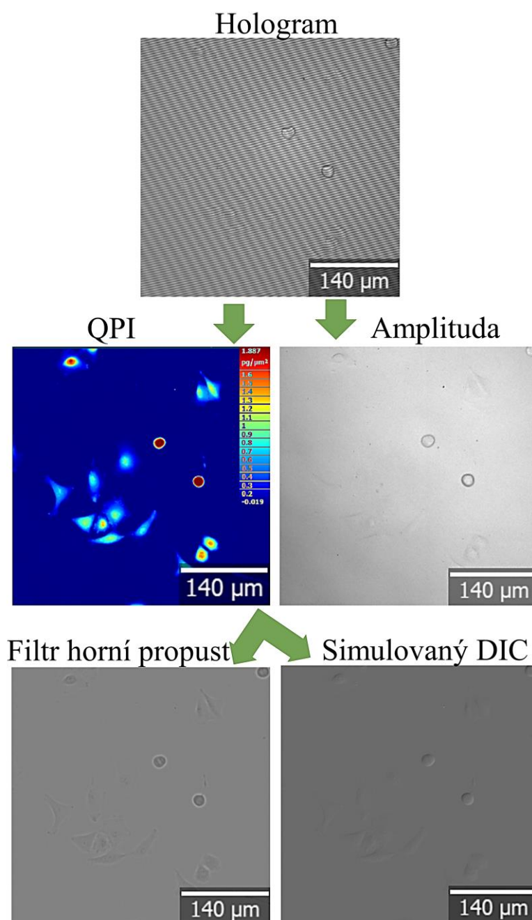
Obrázek č. 5: Multimodální zobrazovací režimy Q-PHASE mikroskopu. K dispozici jsou kromě QPI a amplitudového obrazu i simulovaný DIC nebo horní propust. Objektiv 10x/0,3. Měřítka 140 µm.
