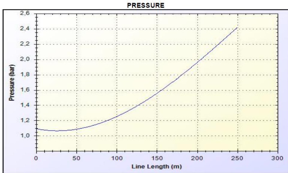
Obrázek 38 - Tlak v závislosti na délce kapkové hadice
