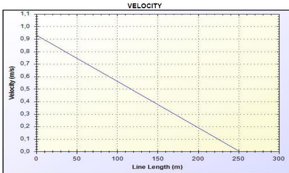
Obrázek 39 - Rychlost kapaliny v závislosti na délce kapkové hadice
