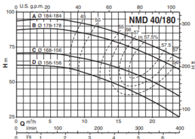
Obrázek 26 - QH charakteristiky navrženého čerpadla
