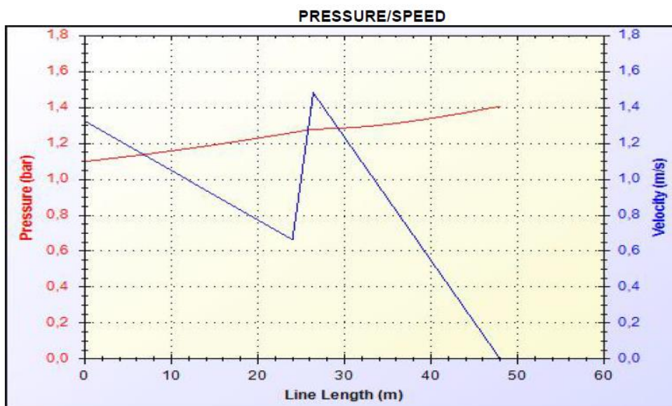
Obrázek 40 - Tlak a rychlost závislá na délce sekčního potrubí
