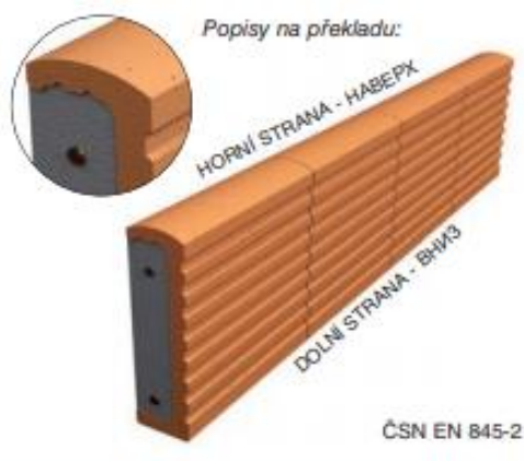
Obr. 4.17 Porotherm překlady KP 7
