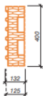
Obr. 4.6 Porotherm 40 P+D ½ K; řez a pohled
