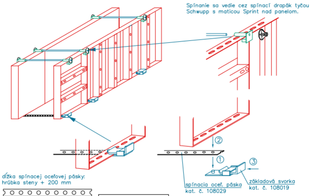
Obr. 6.8 Bednění atiky
