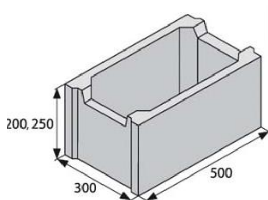
Obr. 4.13 Tvarovky BEST 30; pohled
