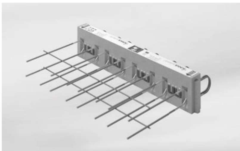
Obr. 4.28 Isokorb Q10S-VV
