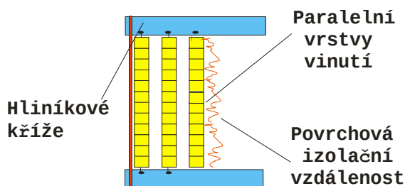
Obr.č.4: Paralelně spojené vrstvy střídavé tlumivky
