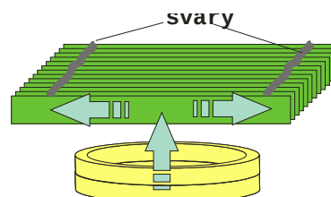
Obr.č.14: Horní spojka magnetického stínění tlumivky při správné orientaci plechů
