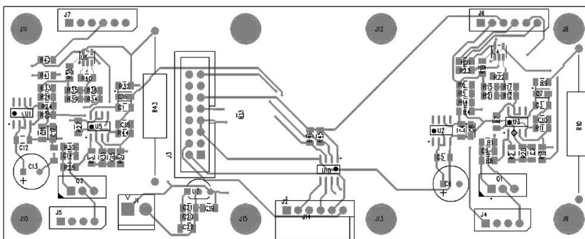
Obr. I.1 Návrh DPS –mainboard. Pohledy TOP, BOTTOM a osazovací výkres
