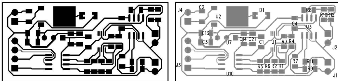
Obr. IV.1 Návrh DPS – ovládání galvozrcátek. Pohledy TOP a osazovací výkres
