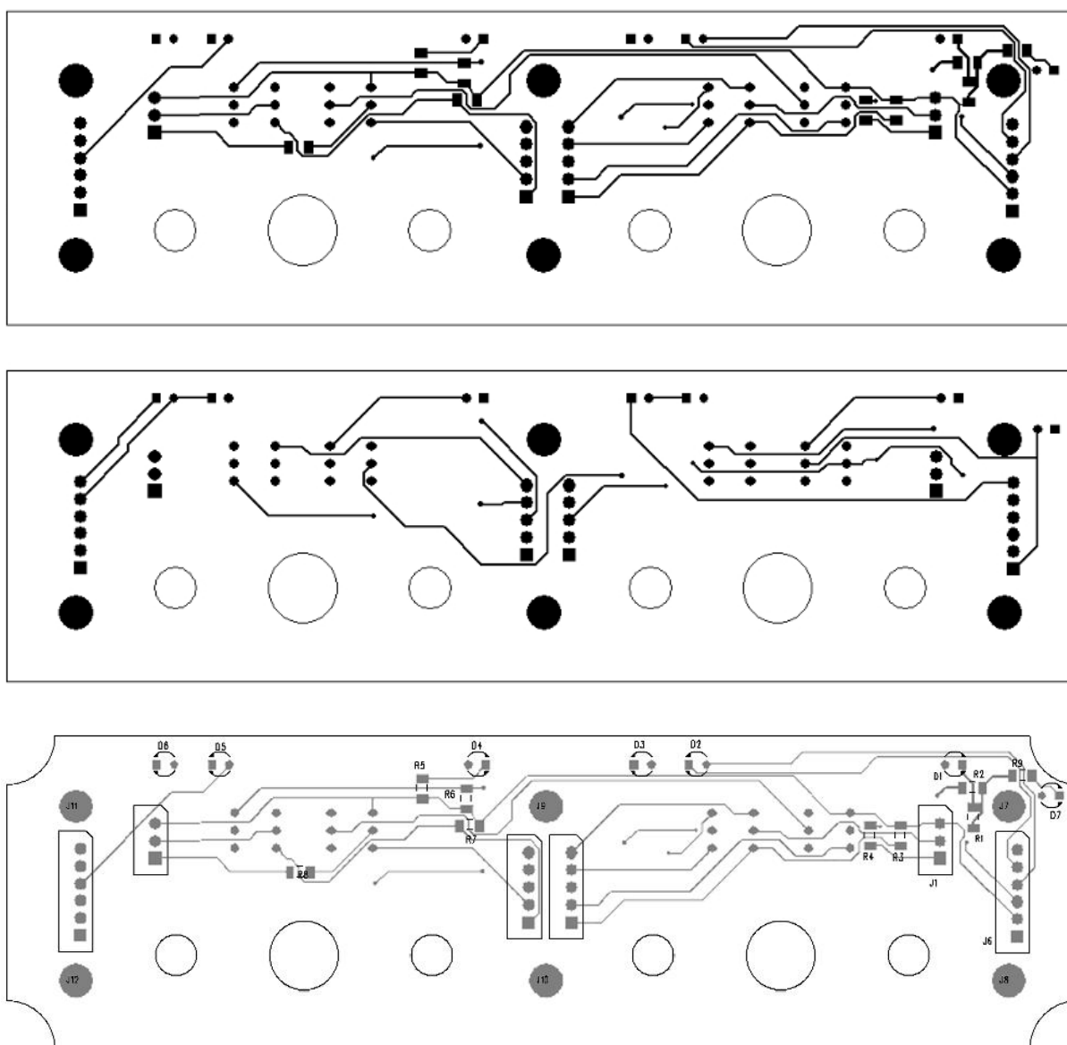
Obr. III.1 Návrh DPS – štítek. Pohledy TOP, BOTTOM a osazovací výkres
