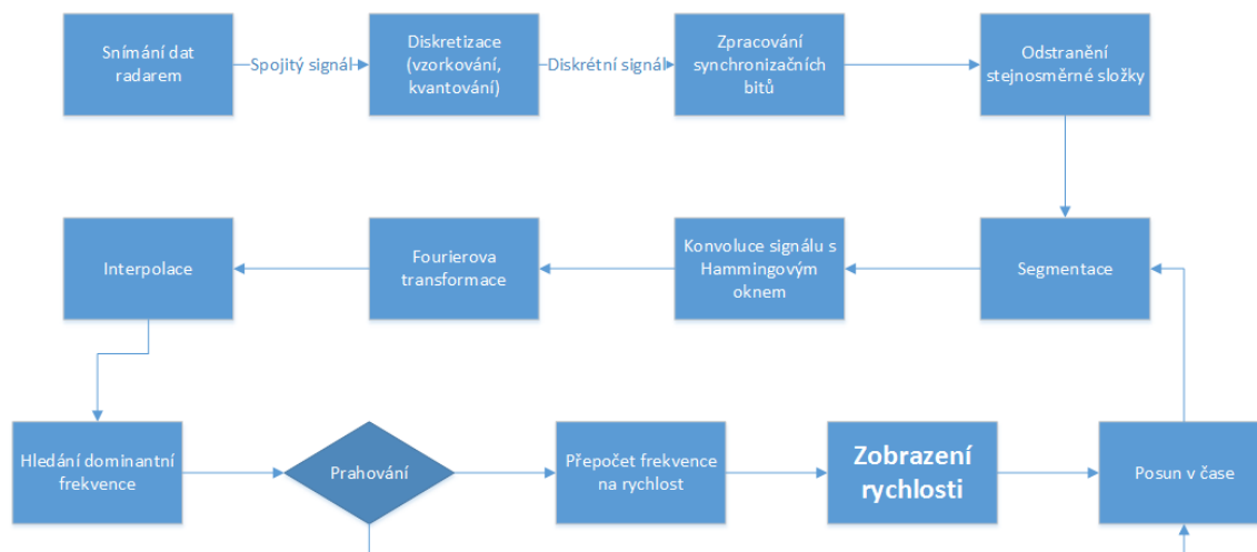
Obrázek 4.1: Procesy v obecném algoritmu
