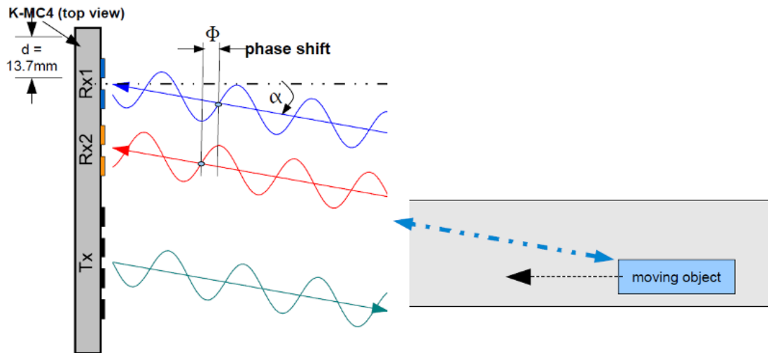
Obrázek 3.6: Měření úhlu radarem KMC4. Zdroj [5]
