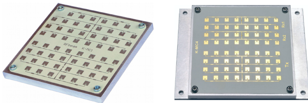
Obrázek 3.3: Fotografie KMC-1 a KMC-4. Zdroj [4] a [5]
