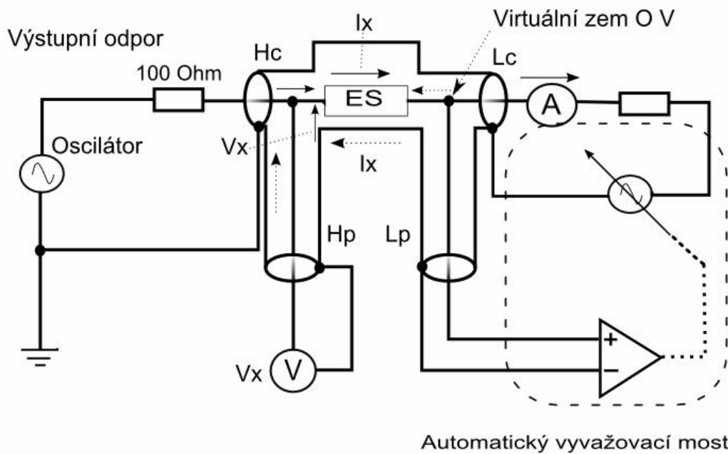
Obr. 3.1 Princip měření přístroje HP 4284A (ES-elektrodotový systém)
