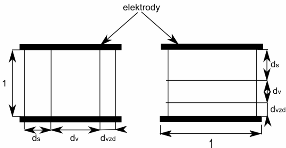
Obr. 2.6 Schematický model vlhkého dielektrika
