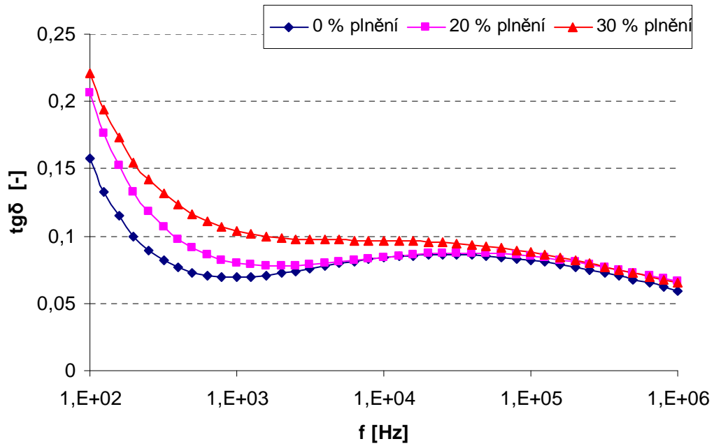
Obr. 3.20 Kmitočtová závislost tg\delta při teplotě 120 °C s relativní vlhkostí 0 % a s plněním jako parametrem
