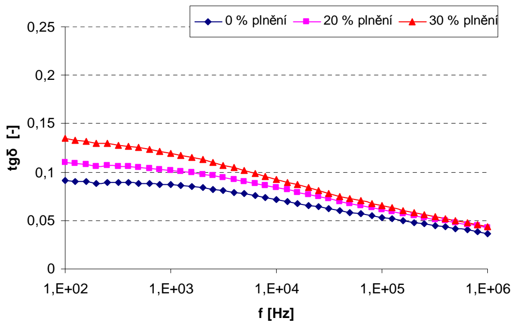
Obr. 3.19 Kmitočtová závislost tg\delta při teplotě 100 °C s relativní vlhkostí 0 % a s plněním jako parametrem
