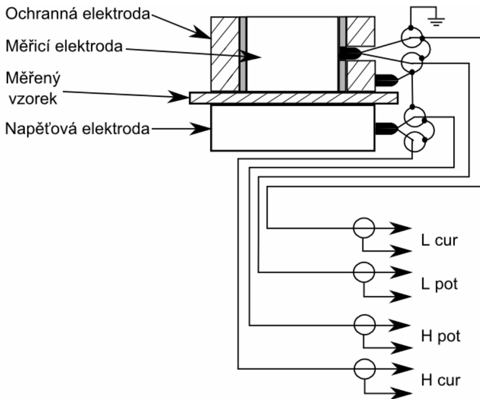
Obr. 3.2 Zapojení elektrodotového systému k HP 4284A z Obr. 3.1
