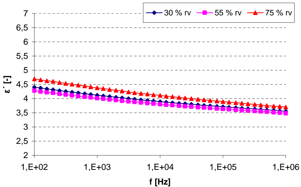
Obr. 3.34 Kmitočtová závislost \epsilon' vzorku plněného 20 % slídou při 24 °C a s relativní vlhkostí jako parametrem
