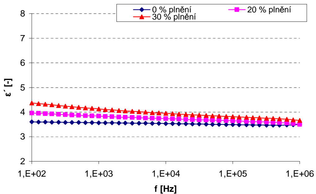
Obr. 3.21 Kmitočtová závislost \epsilon' při teplotě 24 °C s relativní vlhkostí 0 % a s plněním jako parametrem
