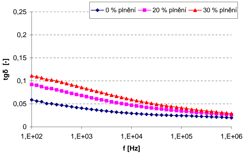
Obr. 3.18 Kmitočtová závislost tg\delta při teplotě 80 °C s relativní vlhkostí 0 % a s plněním jako parametrem
