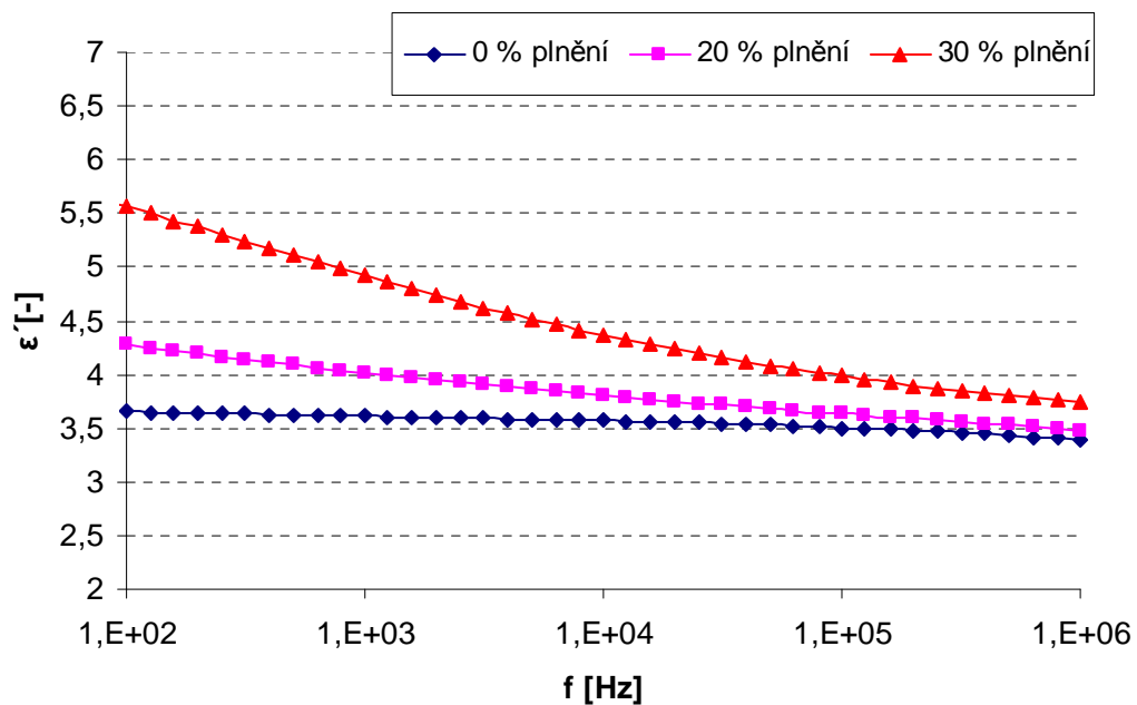
Obr. 3.28 Kmitočtová závislost \epsilon' při teplotě 24 °C s relativní vlhkostí 55 % a s plněním jako parametrem
