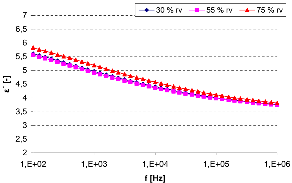
Obr. 3.35 Kmitočtová závislost \epsilon' vzorku plněného 30 % slídou při 24 °C a s relativní vlhkostí jako parametrem
